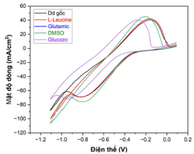
Hình 3: Đường CV của điện dịch anolyt không có và có 2% mol các chất phụ gia khác nhau ở tốc độ quét 3 mV/s trong khoảng điện thế từ -1,1 – 0,1 V
